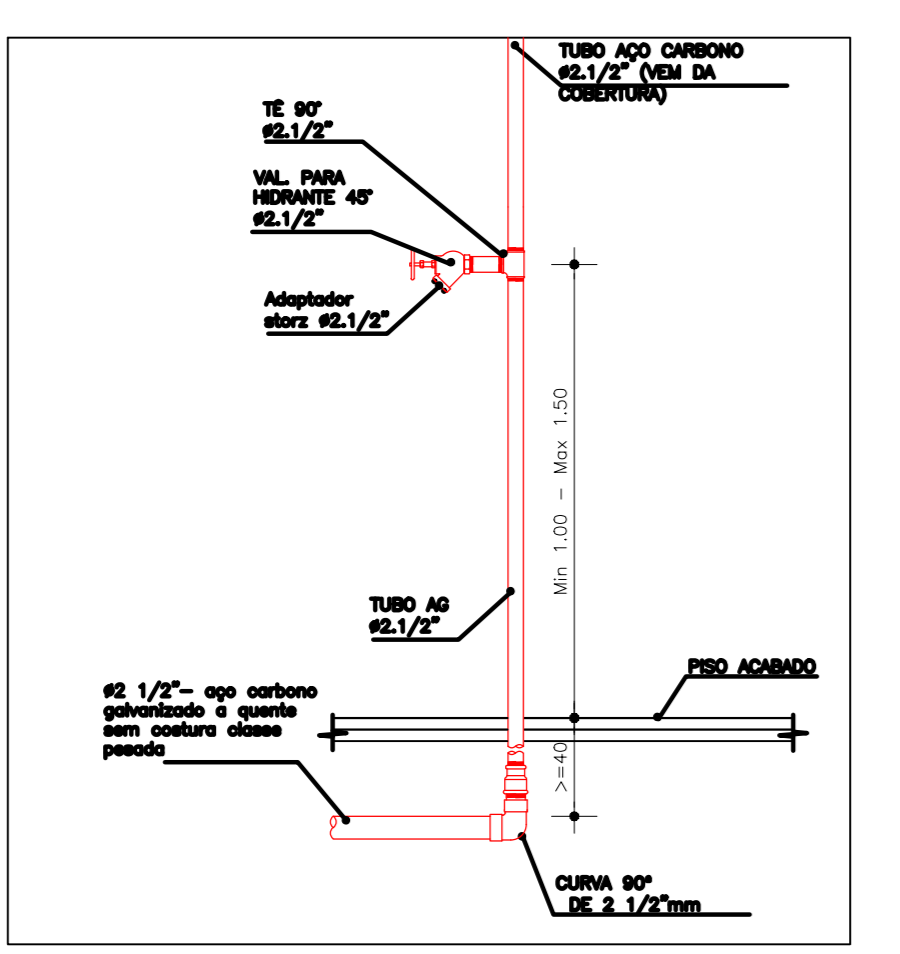
HIDRANTE DE INCÊNDIO PAV. TÉRREO ESCALA: 1:25
