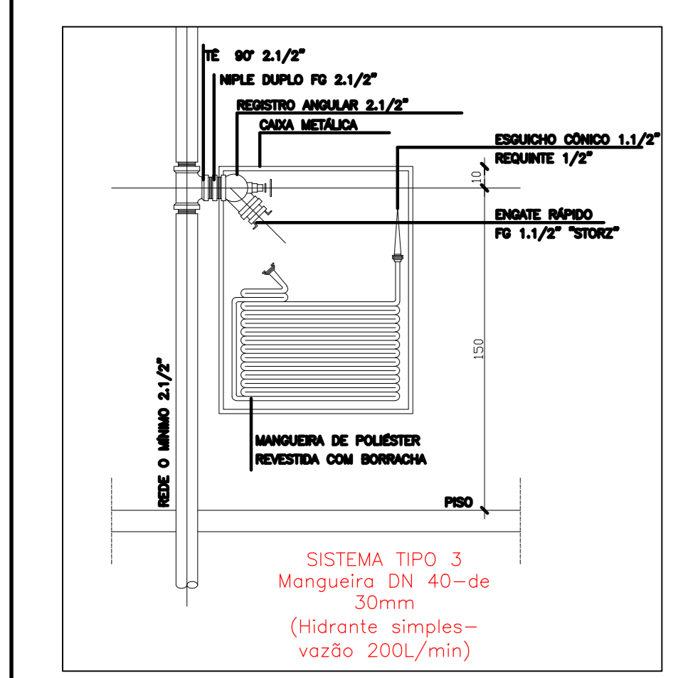
HIDRANTE DE INCÊNDIO PAV. TÉRREO ESCALA: 1:25
